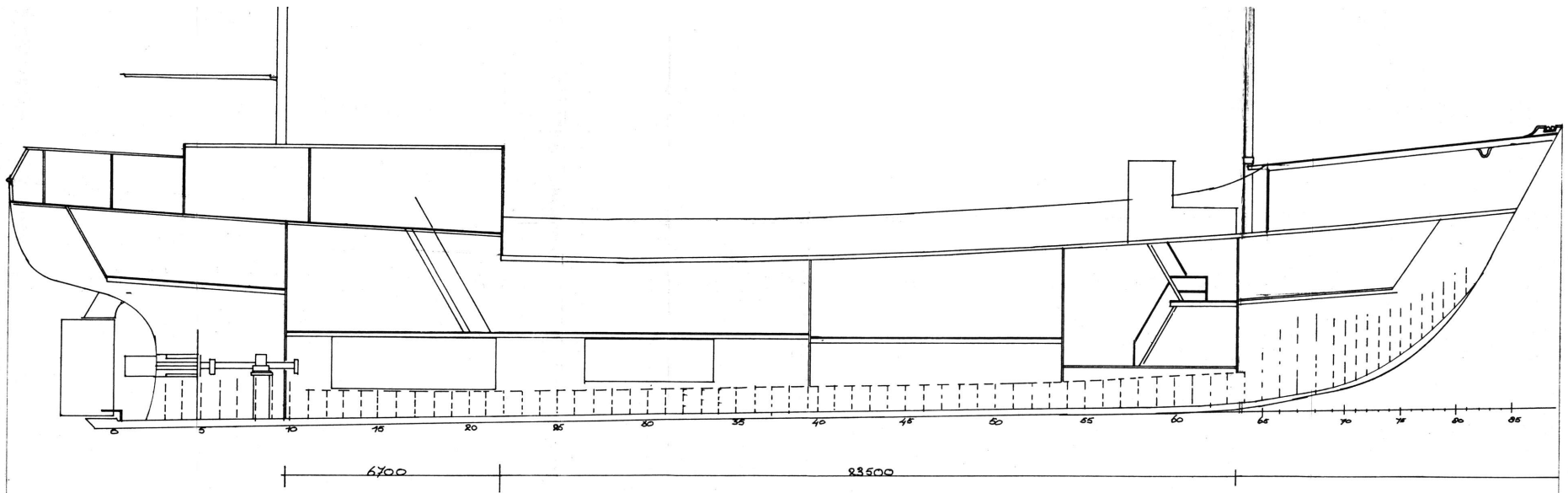
bestaande doorsnede
